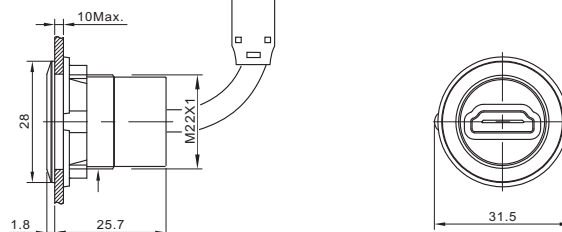
产品描述 : 头部HDMI母/尾部HDMI公 Product Description: HDMI FEMALE/HDMI MALE 线长 : 约60cm Wire Length : About 60cm
